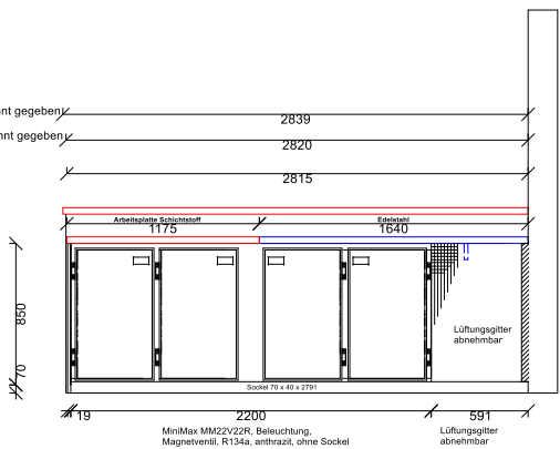
ANSICHT WIRTESEITE
