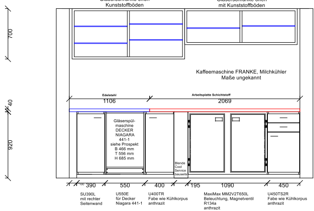
ANSICHT RÜCKTHEKE
